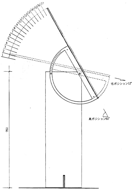
展示台 DETAIL 1:15
